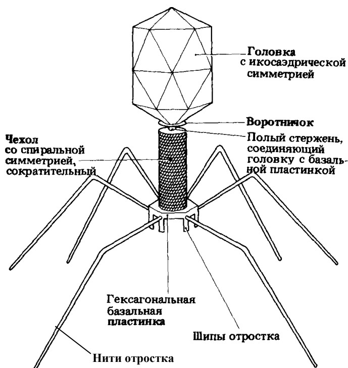
Рис. 3.4. Строение бактериофага.
